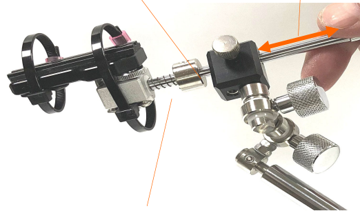
1. スプリング部 をシンプルな構造としました。
